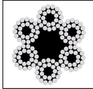
6x24+7
