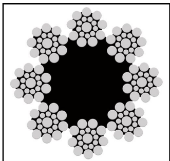
8x19S
