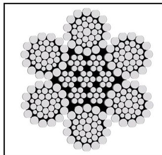
6x36WS IWRC
