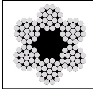
6x19+CF
