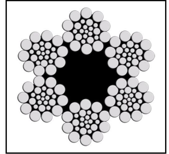
6x26WS
