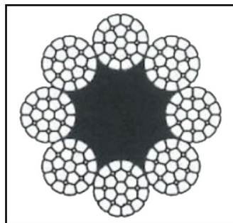
8xFi(25)+FC
